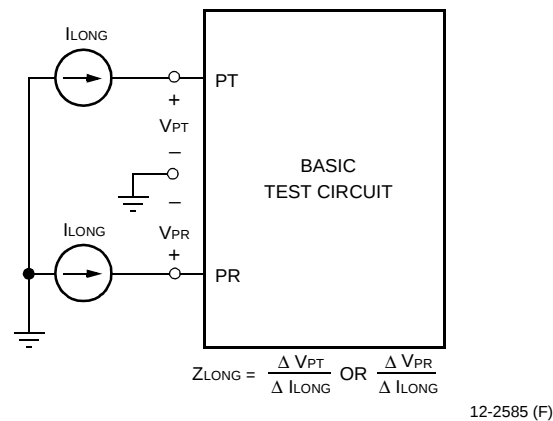
Figure 9. Longitudinal Impedance
